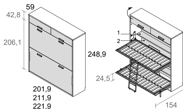
cama horizontal doble con altillo, fondo 59 y altura 248,9
