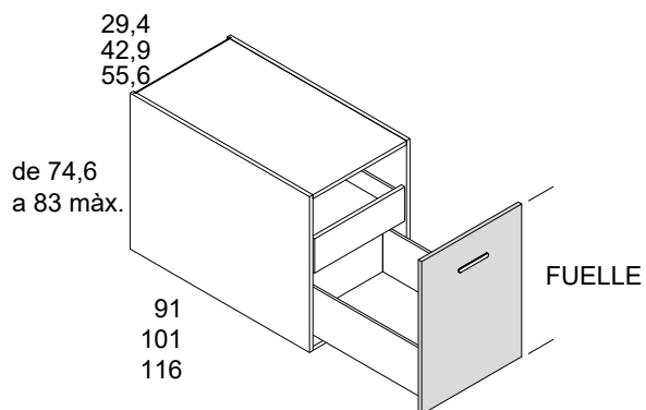
arcón lateral puerta entera - FUELLE -
