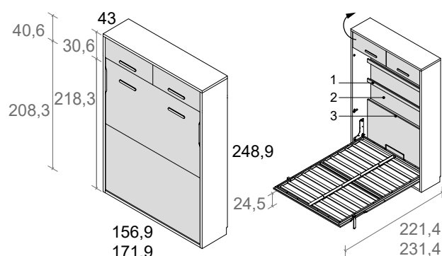
cama vertical con altillo, fondo 43 y altura 248,9
