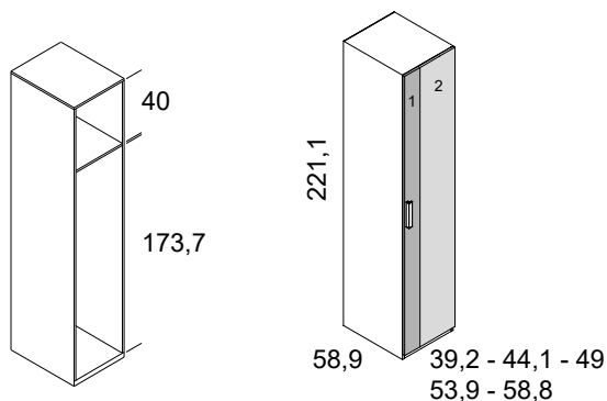
armario 1 puerta derecha con panel vertical
