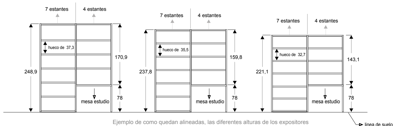
lateral expositor (7 estantes)
