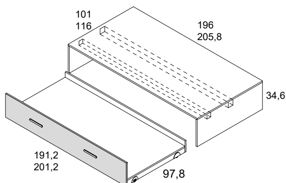
bloc con base y ruedas - 34,6 de alto -
