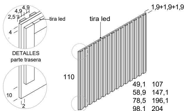
cabezal alistonado con led
