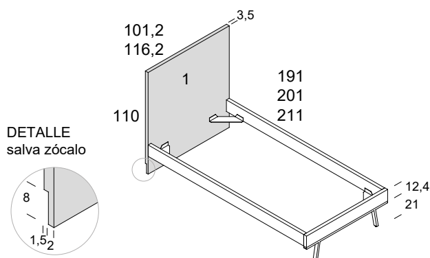
aro y cabezal de melamina con 1 pie metálico
