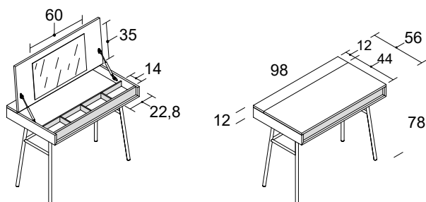
tocador tapa abatible con espejo
