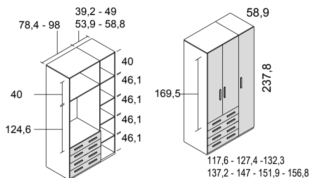
armario 3 puertas y 4 cajones
