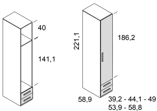
armario 1 puerta derecha y 2 cajones
