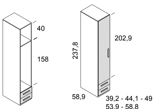
armario 1 puerta izquierda y 2 cajones
