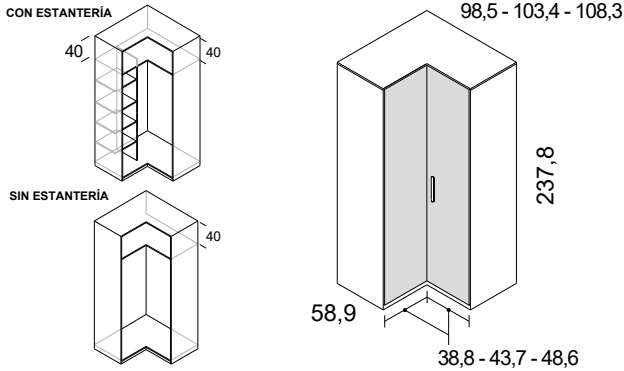
armario rincón escuadra 2 puertas rectas
