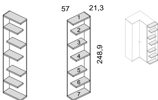
estantería terminal recta con estantes desiguales
