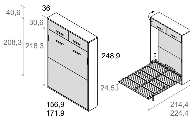
cama vertical con altillo, fondo 36 y altura 248,9
