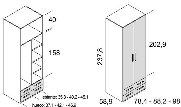
armario 2 puertas y 2 cajones, interior con divisor y estantería derecha
