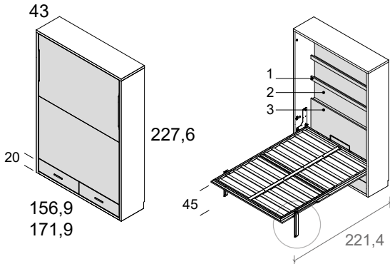
cama vertical simple sin sofá con patas altas y 2 cajones frontales
