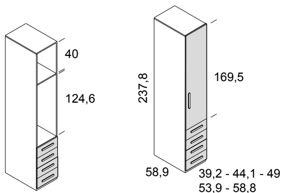
armario 1 puerta derecha y 4 cajones
