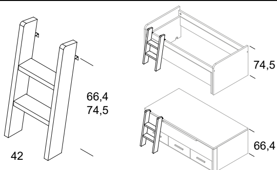
escalera móvil para compactas
