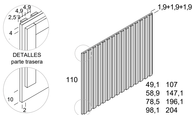
cabezal alistonado sin led
