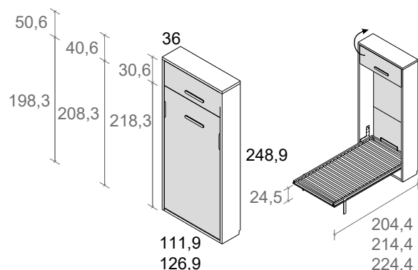
cama vertical con altillo, fondo 36 y altura 248,9
