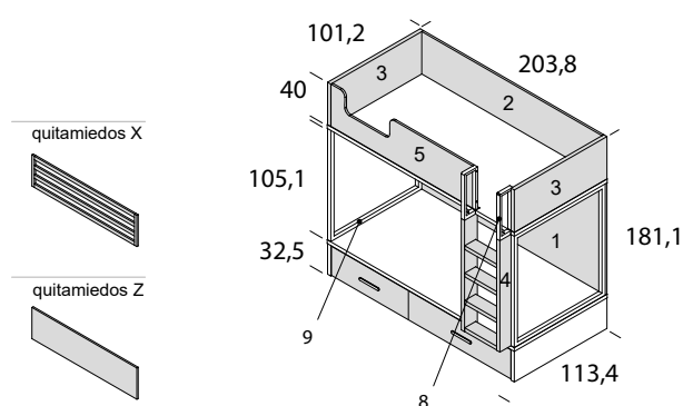
litera con cama inferior + 2 cajones nido con ruedas
