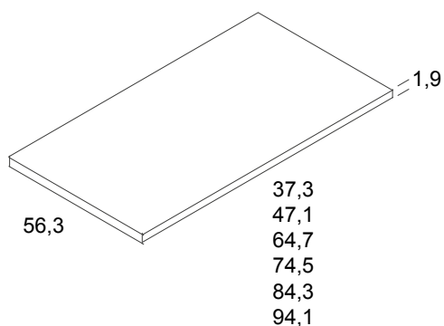
estante interior para armarios puertas correderas interiores y colgadas
