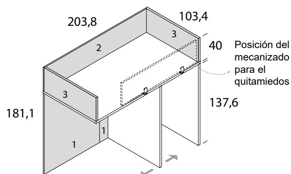
tren superior derecho (bajos 137,6)
