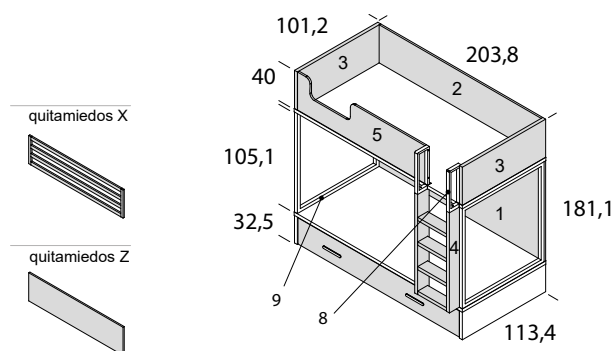
litera con cama inferior + tapa con arrastre
