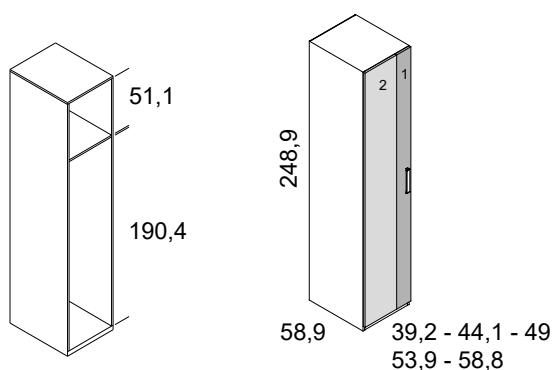
armario 1 puerta izquierda con panel vertical
