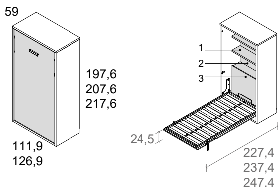
cama vertical sin altillo, fondo 59
