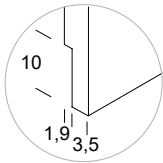
DETALLE salva zócalo
