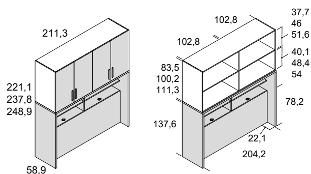
Puente con arcón y estantería para cama de 190
