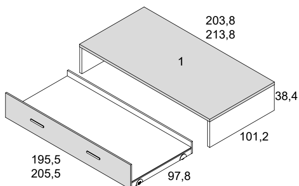
nido con base y ruedas
