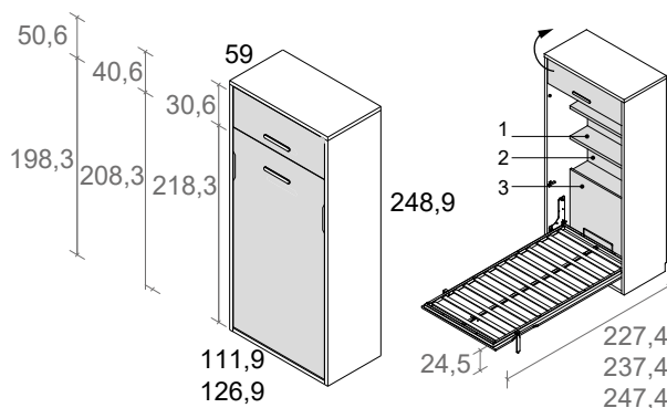
cama vertical con altillo, fondo 59 y altura 248,9
