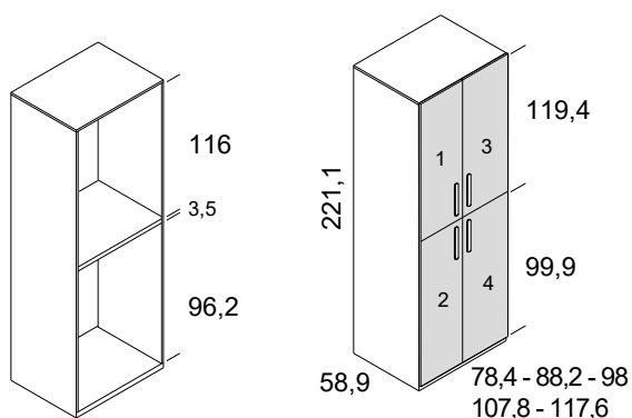
armario estacional 4 puertas
