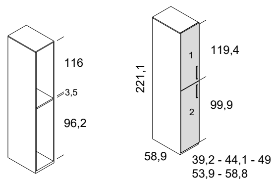
armario estacional 2 puertas izquierdas
