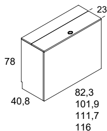
DETALLE salva zócalo
