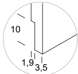
DETALLE salva zócalo
