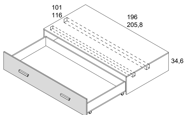
bloc cama cajón con ruedas - 34,6 de alto -
