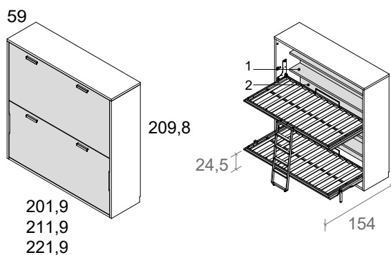
cama horizontal doble sin altillo, fondo 59
