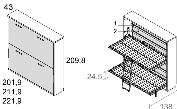
cama horizontal doble sin altillo, fondo 43
