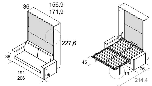
cama vertical simple con sofá canapé, fondo 36
