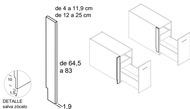
tapeta - FUELLE - para arcones
