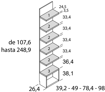
Estantería FUELLE para alinear con las camas abatibles
