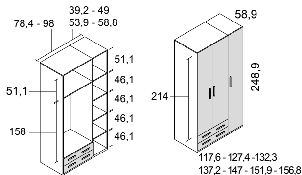
armario 3 puertas y 2 cajones izquierda
