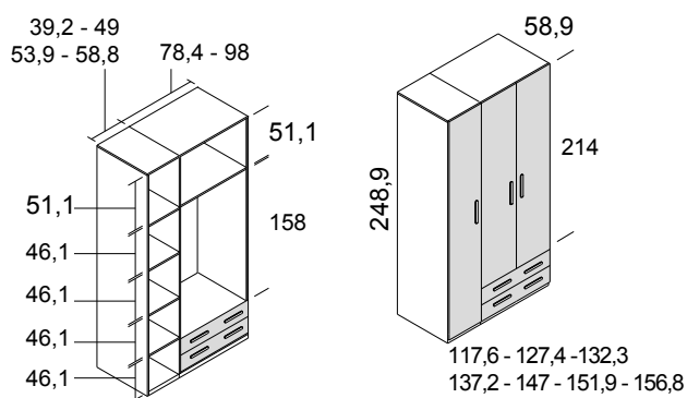
armario 3 puertas y 2 cajones derecha
