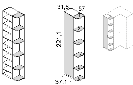
armario terminal zapatero curvo puerta recta izquierda
