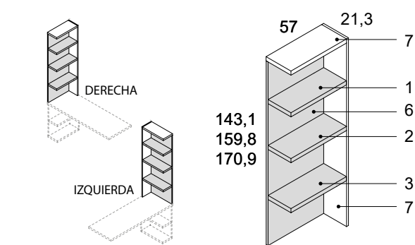
estantería terminal para mesa estudio
