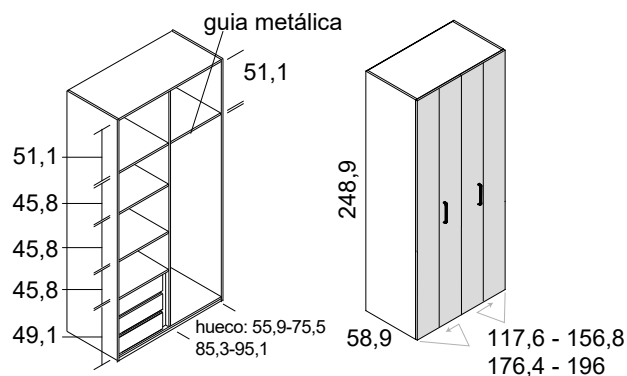
armario 2 puertas plegables
