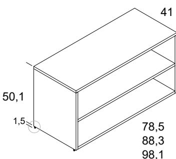
DETALLE taco (opcional)
