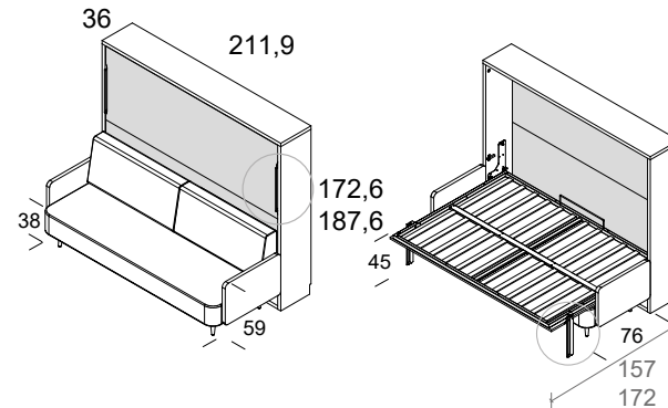
camas horizontal simple con sofá nórdico fondo 36
