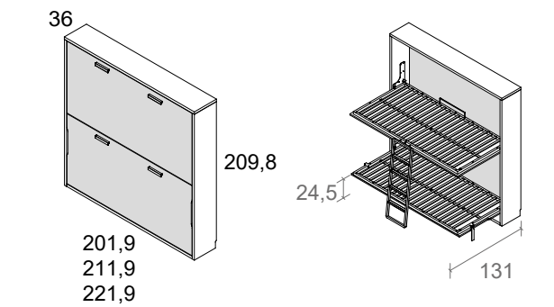
cama horizontal doble sin altillo, fondo 36
