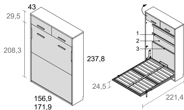
cama vertical con altillo, fondo 43 y altura 237,8
