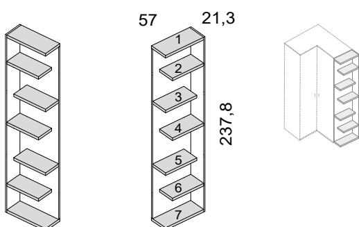
estantería terminal recta estantes desiguales
