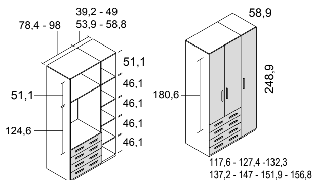
armario 3 puertas y 4 cajones izquierda
