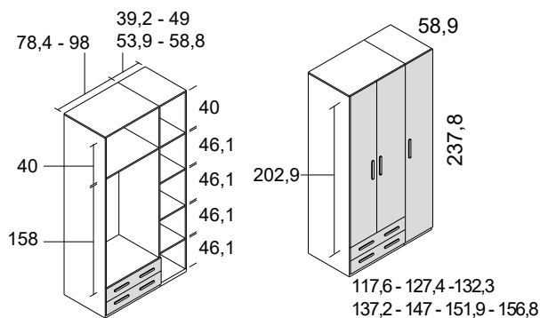
armario 3 puertas y 2 cajones
