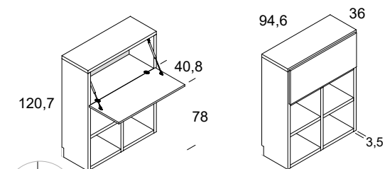
DETALLE salva zócalo
