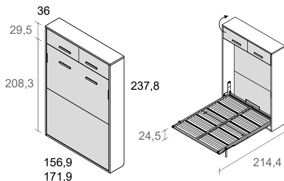
cama vertical con altillo, fondo 36 y altura 237,8
