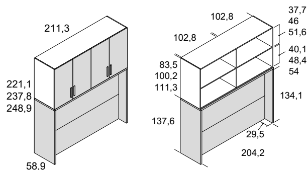
Puente con estructura soporte diáfana para cama de 190
