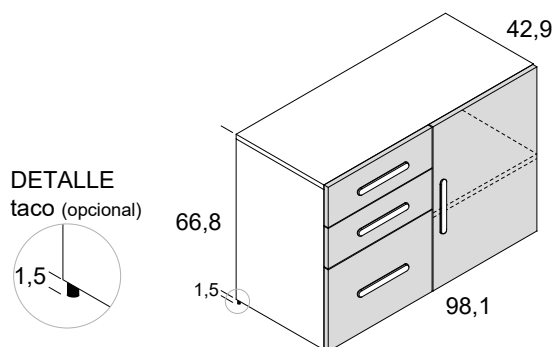
módulo 2 cajones y contenedor + puerta derecha
