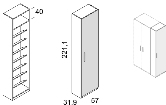
armario lateral zapatero derecho con puerta entera
