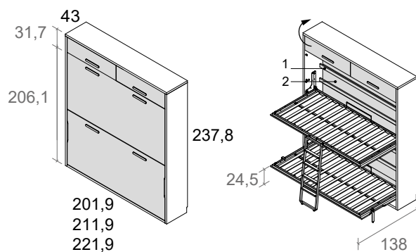
cama horizontal doble con altillo, fondo 43 y altura 237,8
