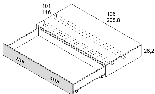
bloc cama cajón con ruedas - 26,2 de alto -
