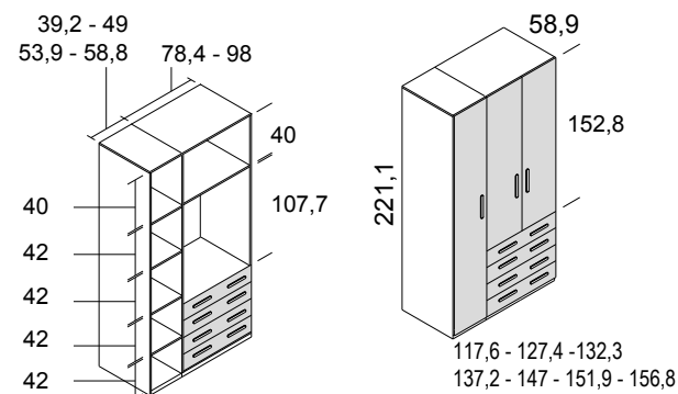
armario 3 puertas y 4 cajones derecha
