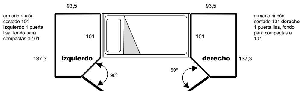
armario rincón derecho, costado 101, con 1 puerta
