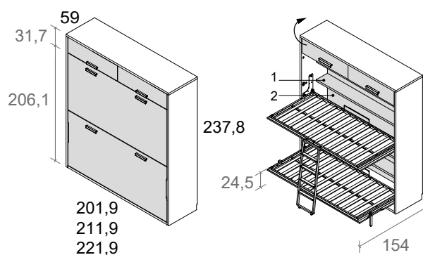
cama horizontal doble con altillo, fondo 59 y altura 237,8
