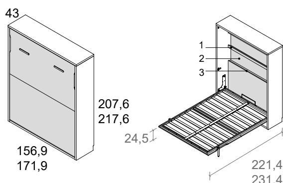
cama vertical sin altillo, fondo 43
