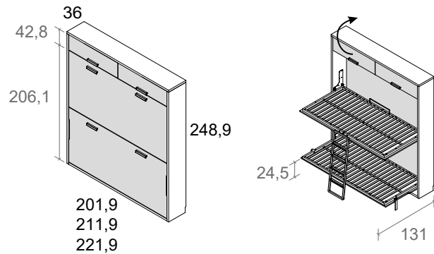
cama horizontal doble con altillo, fondo 36 y altura 248,9
