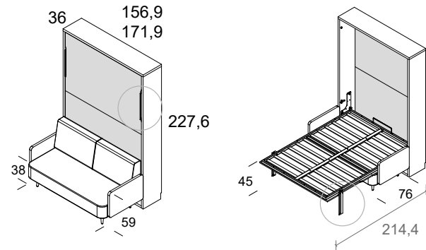
camas vertical simple con sofá nórdico, fondo 36
