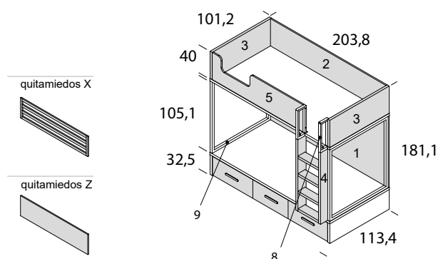
litera con cama inferior + cajonera de 3 cajones de 24,7
