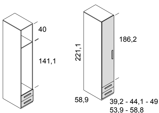
armario 1 puerta izquierda y 2 cajones
