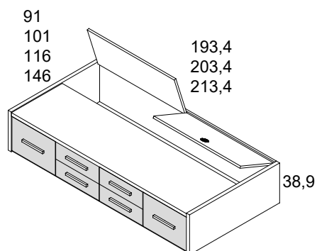
compacta arcón con 4 cajones de 16,4 y 2 contenedores de 33,1
