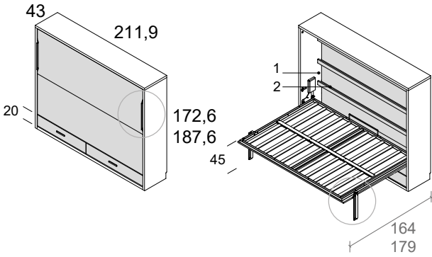
cama horizontal simple sin sofá con patas altas y 2 cajones frontales
