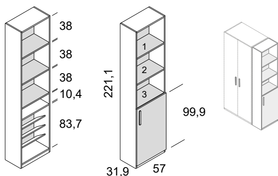
armario lateral zapatero derecho con puerta y estantes
