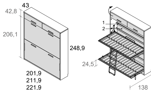
cama horizontal doble con altillo, fondo 43 y altura 248,9
