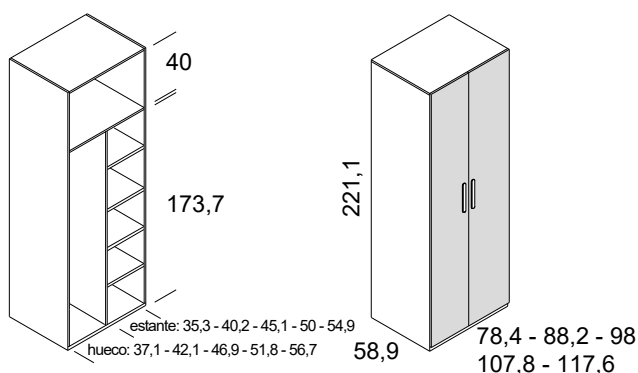
armario 2 puertas con divisor y estantería derecha hasta el bajo.
