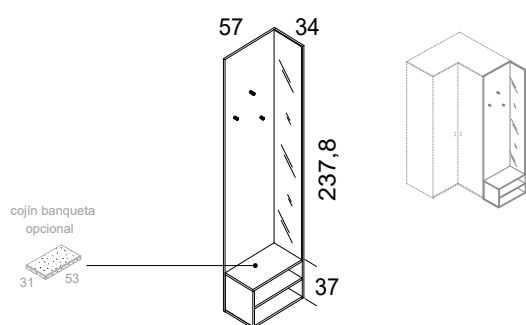
estantería terminal derecha con espejo y colgadores
