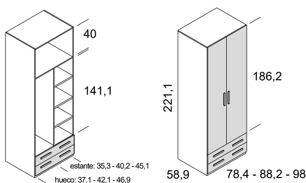
armario 2 puerta y 2 cajones, interior con divisor y estantería derecha
