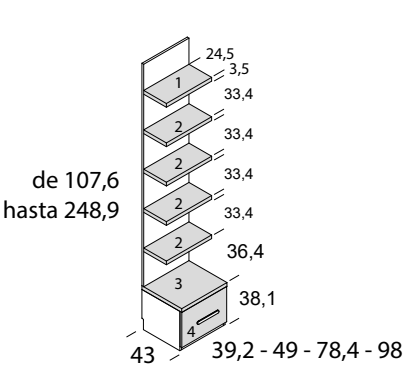
estantería con contenedor FUELLE para alinear con las camas abatibles
