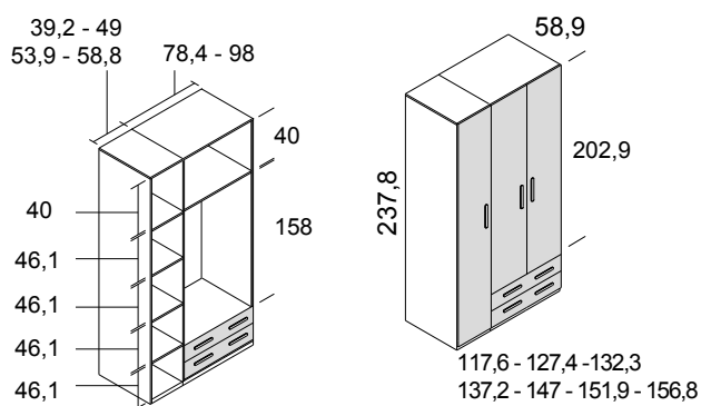
armario 3 puertas y 2 cajones
