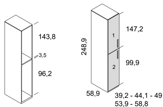
armario estacional 2 puertas izquierdas
