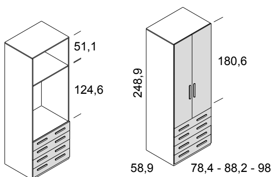
armario 2 puertas y 4 cajones
