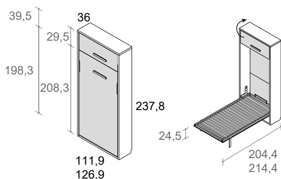
cama vertical con altillo, fondo 36 y altura 237,8
