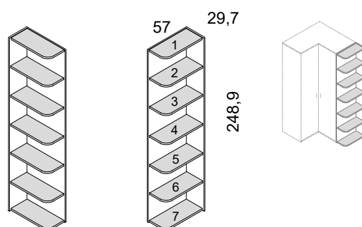
estantería terminal curva
