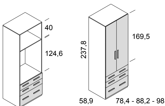
armario 2 puertas, 2 cajones y 1 contenedor
