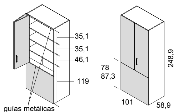
armario puerta plegable izquierda
