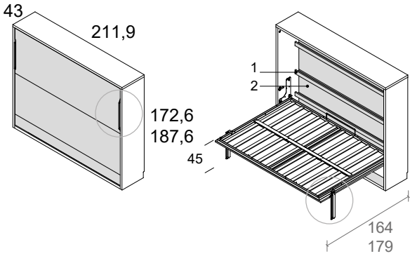
cama horizontal simple sin sofá con patas altas
