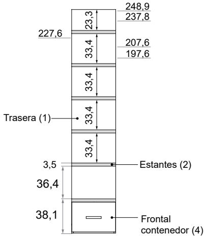
Alturas de camas abatibles VERTICALES
