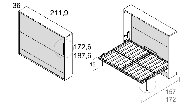
cama horizontal simple sin sofá con patas altas
