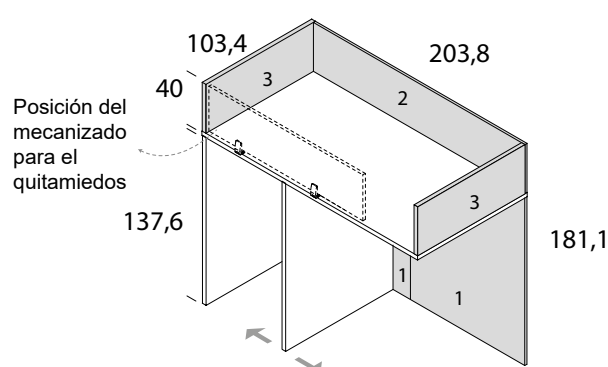
tren superior izquierdo (bajos 137,6)
