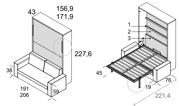
cama vertical simple con sofá canapé, fondo 43
