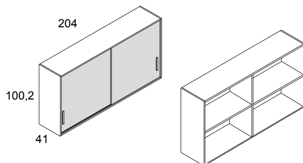
punte 2 puertas correderas
