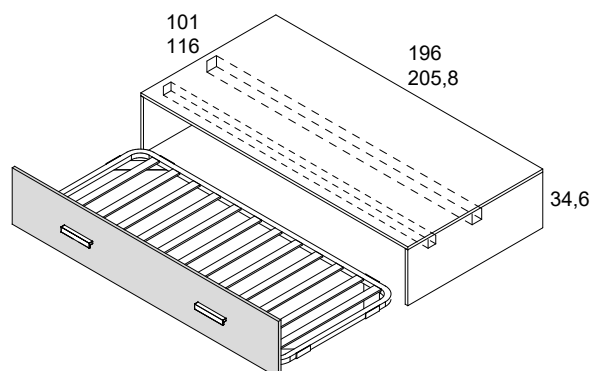
bloc tapa con arrastre - 34,6 de alto -
