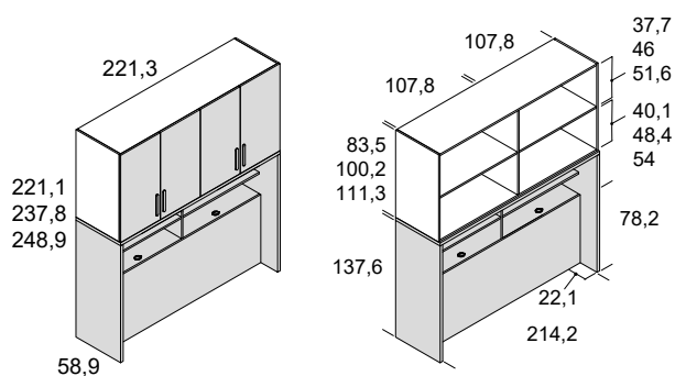
Puente con arcón y estantería para cama de 200
