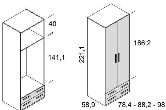
armario 2 puertas y 2 cajones
