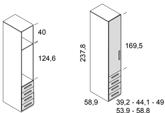
armario 1 puerta izquierda y 4 cajones
