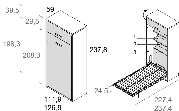
cama vertical con altillo, fondo 59 y altura 237,8
