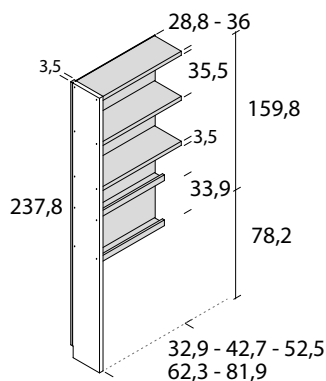
DETALLE salva zócalo
