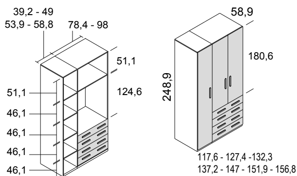
armario 3 puertas y 4 cajones derecha
