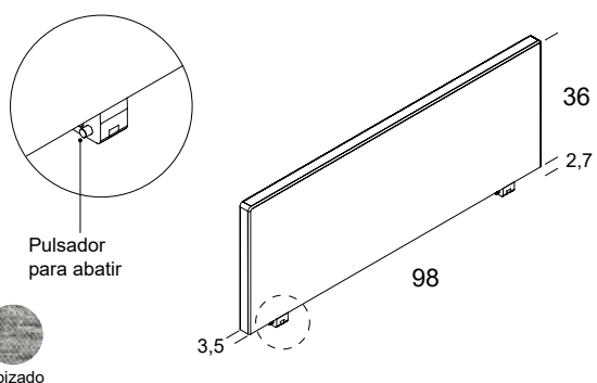
quitamiedos tapizado RECTO para base
