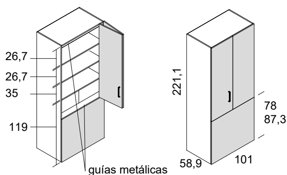
armario puerta plegable derecha
