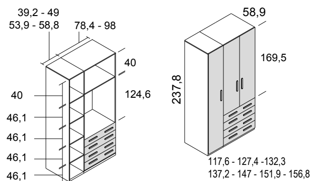
armario 3 puertas y 4 cajones
