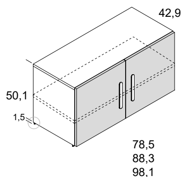
DETALLE taco (opcional)
