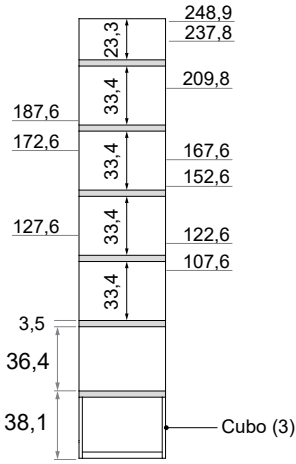
Alturas de camas abatibles HORIZONTALES
