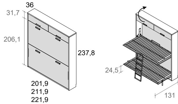
cama horizontal doble con altillo, fondo 36 y altura 237,8
